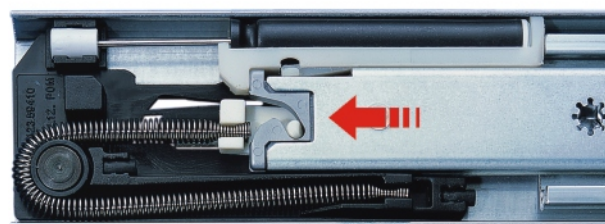
Sortie totale avec "Soft Control" à l'enclenchement
